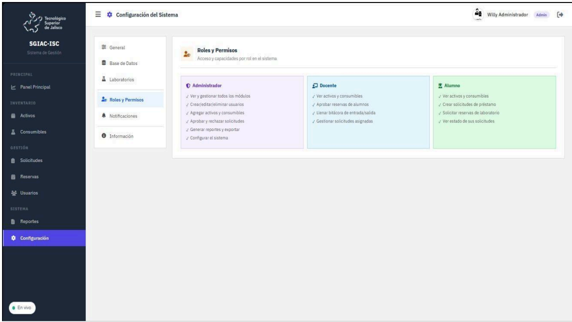
Imagen 11.18.8.4.1 – Pantalla de Roles y Permisos del sistema, donde se visualizan de forma comparativa las capacidades de cada rol: Administrador, Docente y Alumno.
